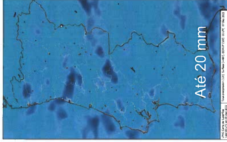
Precipitação 12-24UTC
