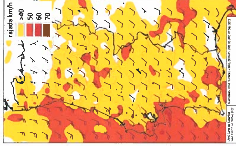
Vento/Rajada 15UTC
