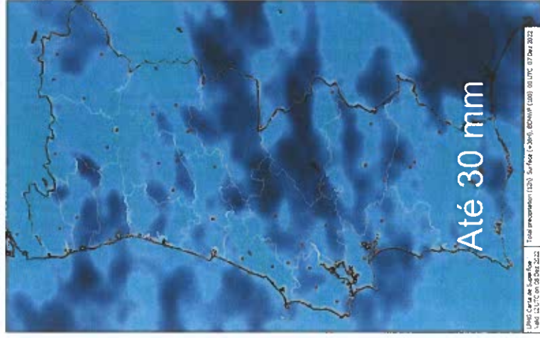
Precipitação 00-12UTC
