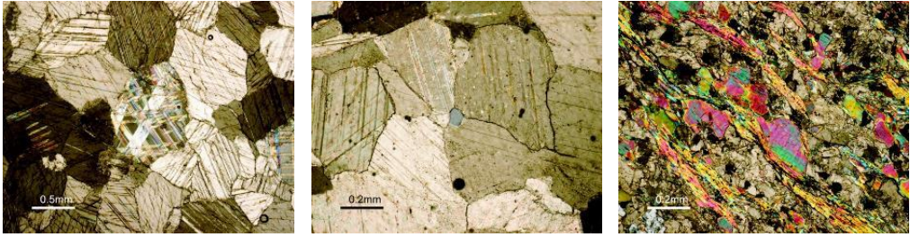
Fig. 4 – Imagens ao microscópio petrográfico do mármore Estremoz Creme. À esquerda e ao centro textura granoblástica praticamente monominerálica equidimensional. Este é o aspecto normal quando a secção de corte coincide com o corte “a favor”. Na figura do meio ao centro destaca-se um pequeno cristal de quartzo entre os cristais de calcite. Na imagem da direita representa-se um nível metavulcânico com textura orientada, nematoblástica e poliminerálicas (quartzo, sericite, moscovite, anfíbola e minerais opacos (secção obtida no corte “ao contra”).
