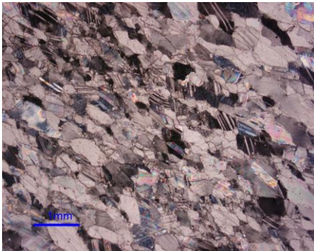
Fig. 5 – Imagens ao microscópio petrográfico do mármore “Azul Lagoa” em secção “a favor”, à esquerda em cima e ao contra”, à esquerda em baixo. Em cima ilustra-se uma inclusão fluída aprisionada no mármore durante o processo metamórfico de recristalização da rocha. Estas inclusões funcionam como geotermómetros e geobarómetros naturais permitindo estimar a temperatura e a pressão a que o metamorfismo ocorreu.
