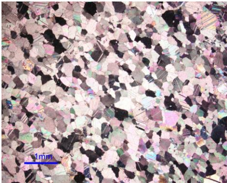
Fig. 4 – Imagens ao microscópio petrográfico do mármore Estremoz Creme. À esquerda e ao centro textura granoblástica praticamente monominerálica equidimensional. Este é o aspecto normal quando a secção de corte coincide com o corte “a favor”. Na figura do meio ao centro destaca-se um pequeno cristal de quartzo entre os cristais de calcite. Na imagem da direita representa-se um nível metavulcânico com textura orientada, nematoblástica e poliminerálicas (quartzo, sericite, moscovite, anfíbola e minerais opacos (secção obtida no corte “ao contra”).
