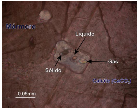
Fig. 5 – Imagens ao microscópio petrográfico do mármore “Azul Lagoa” em secção “a favor”, à esquerda em cima e ao contra”, à esquerda em baixo. Em cima ilustra-se uma inclusão fluída aprisionada no mármore durante o processo metamórfico de recristalização da rocha. Estas inclusões funcionam como geotermómetros e geobarómetros naturais permitindo estimar a temperatura e a pressão a que o metamorfismo ocorreu.
